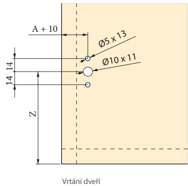
Vrtání dveří
