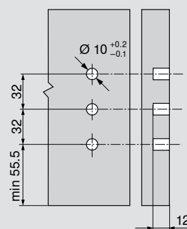
Rozměry pro vyvrtání otvorů u čela pro EXPANDO
