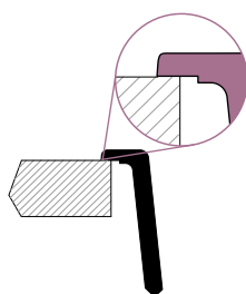
Horní uložení montáž bez příchytok
