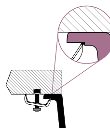
Spodní uložení montáž s příchytkami
