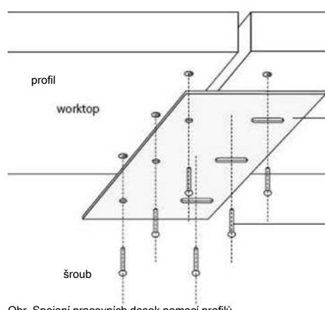
Obr. Spojení pracovních desek pomocí profilů.
