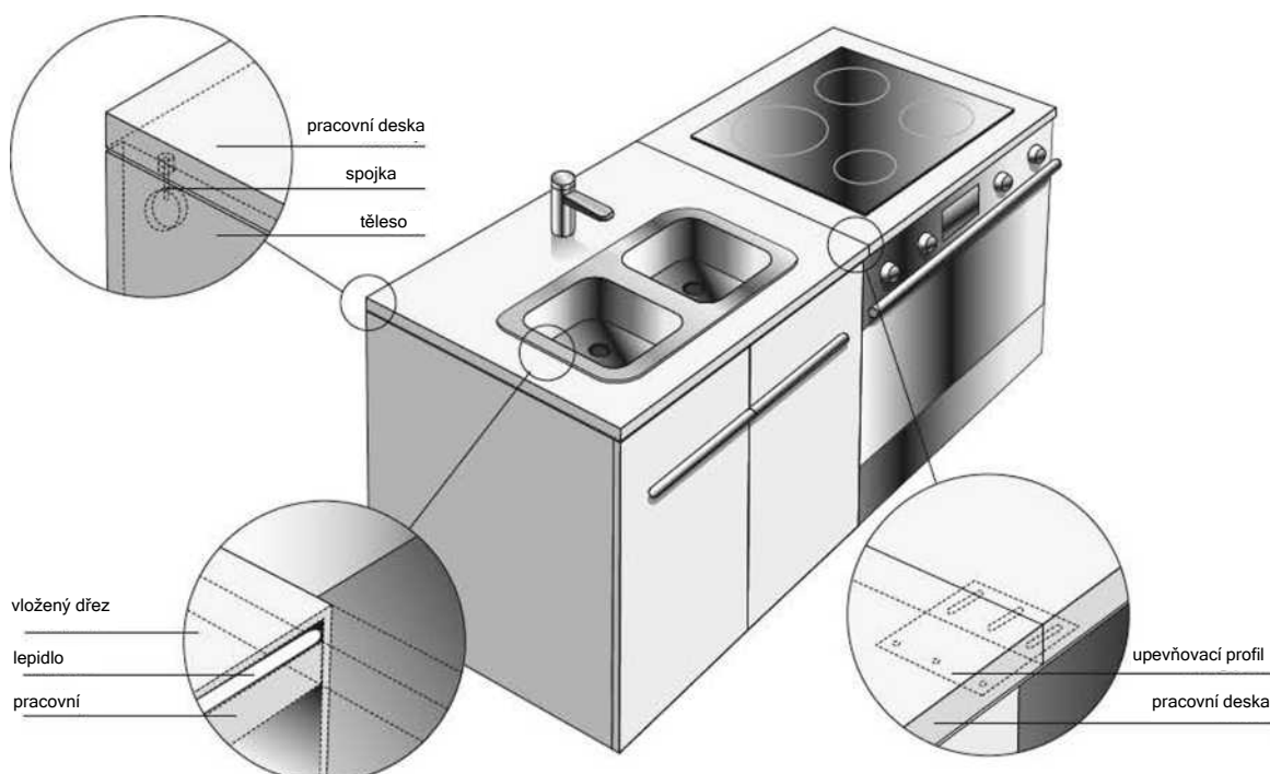
Obr. Instalace nábytku vyrobeného z panelů Krono Compact - na příkladu kuchyně.
