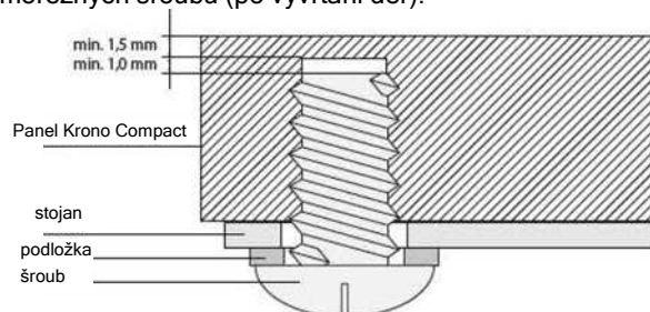
Obr. Upevnění pracovní desky na stojany.
