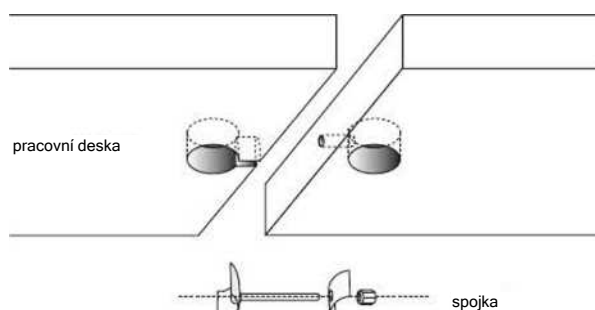
Obr. Spojení pracovních desek pomocí spojek.
