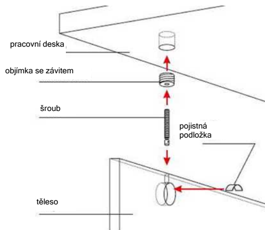
Obr. Upevnění pracovní desky z dřevotřísky.
